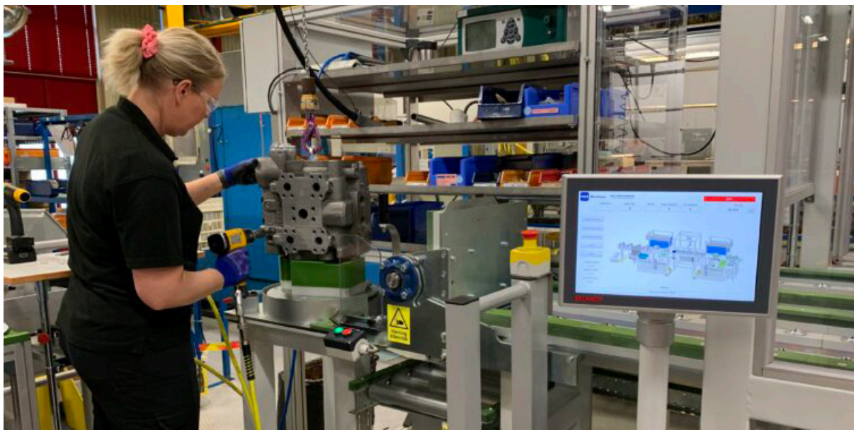
Cobot-produktionslina som levererats till Parker Hannifin
